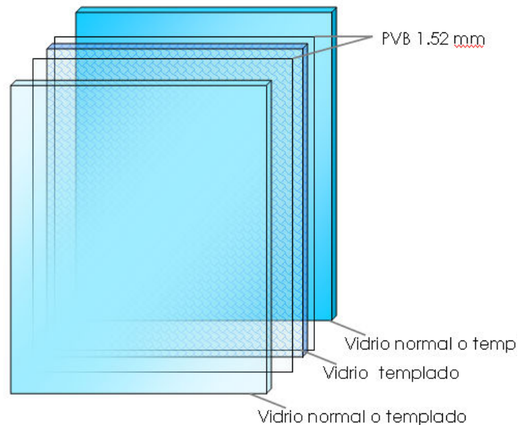
Figura 2. Configuración de un vidrio craquelado.
