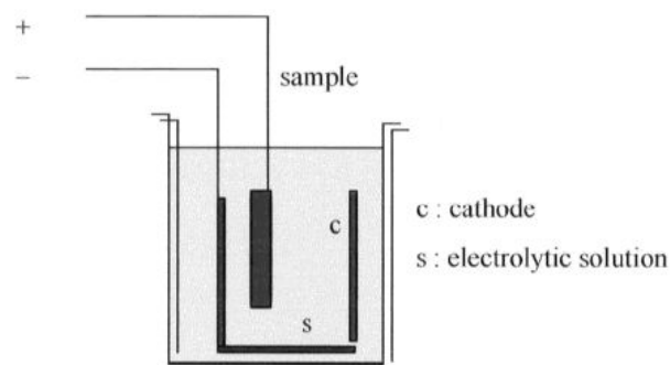
Imagen 1. Representación esquemática del proceso de electrólisis
