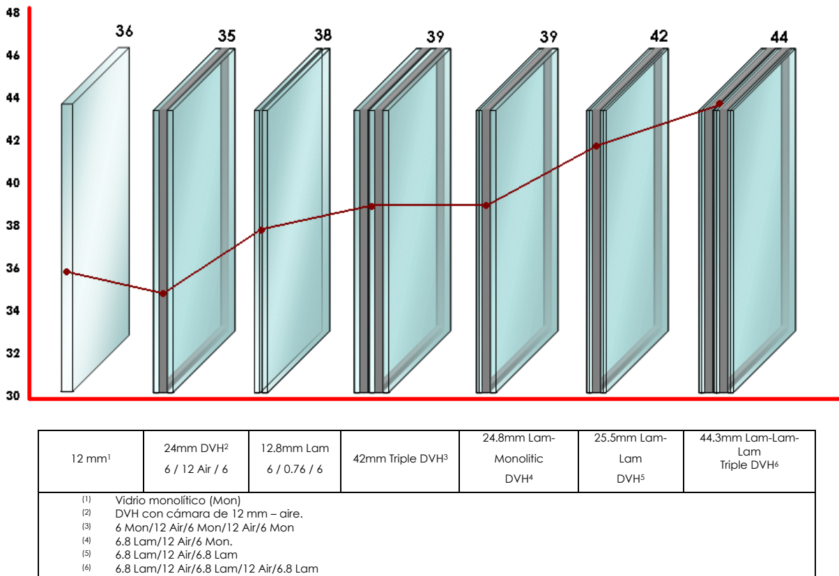
Gráfico 1. Valores de STC para diferentes configuraciones de vidrio
